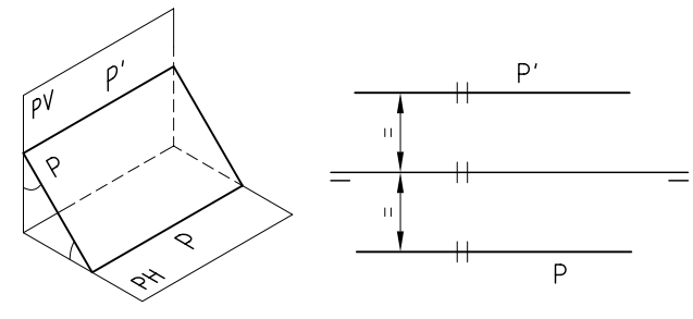
Perpendicular al segundo bisector
