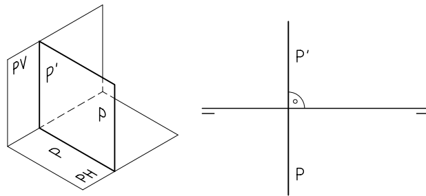
Perpendicular al plano horizontal (proyectante horizontal)
