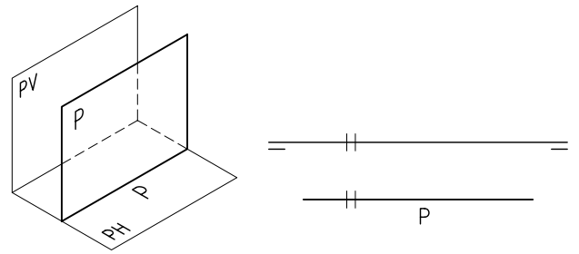
Paralelo al Plano Vertical
