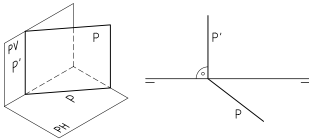
Perpendicular al plano horizontal (proyectante horizontal)
