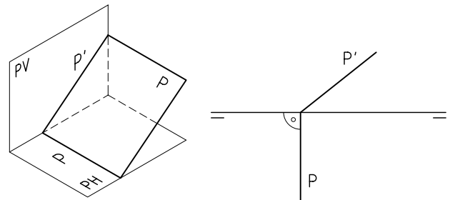
Perpendicular al Plano Vertical (proyectante vertical)
